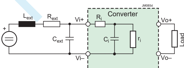
Fig. 2 Input configuration
