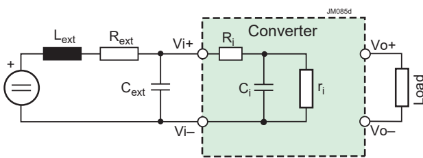
Fig. 2 Input configuration
