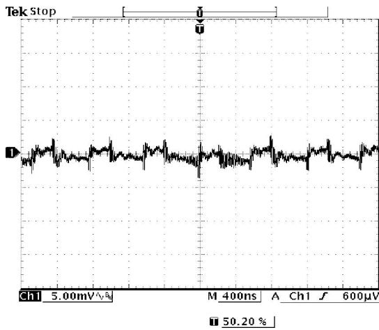
VRP4-C0E1A0 12Vdc input, VID=0x52, Iout=70A, PSI#=1
