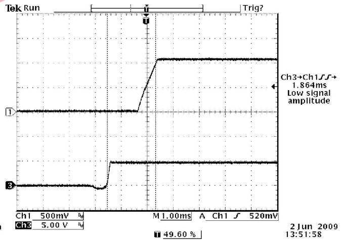
VID=0x52, Vin=12V, Iout=0A CH 1: Vout CH 3: IOUTEN
